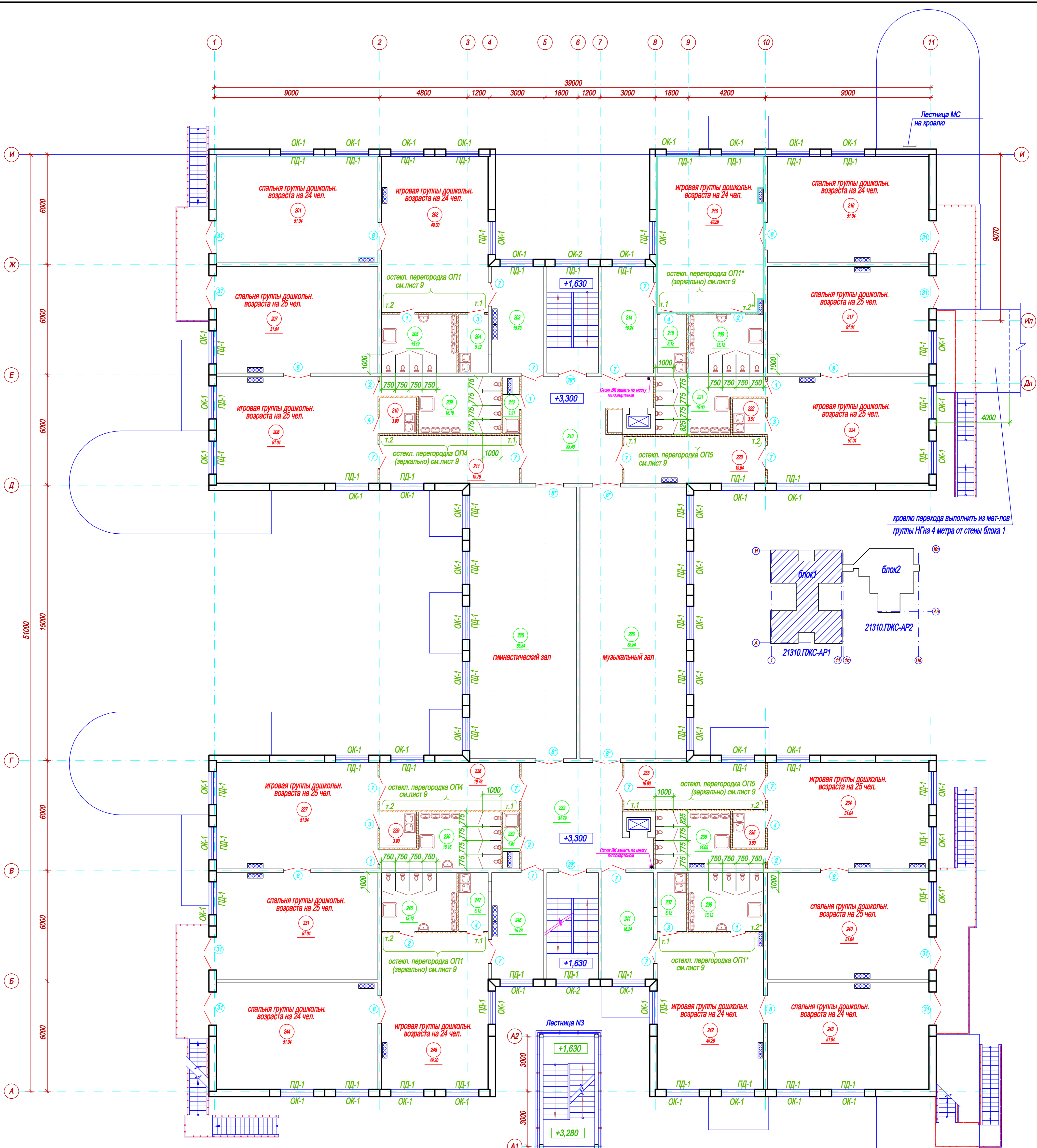
Экспликация помещений 2 этажа
